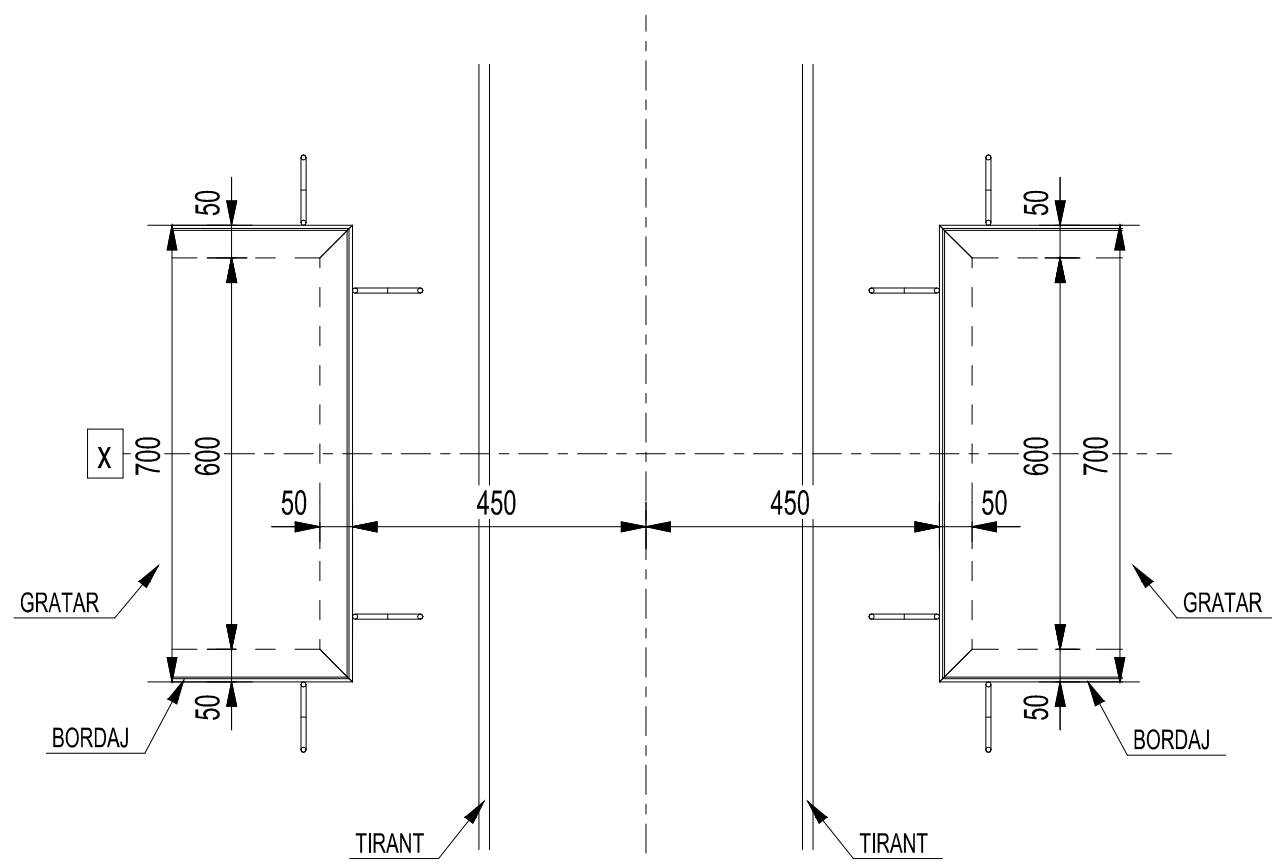
DETALIU NOD CURENT 1:15
